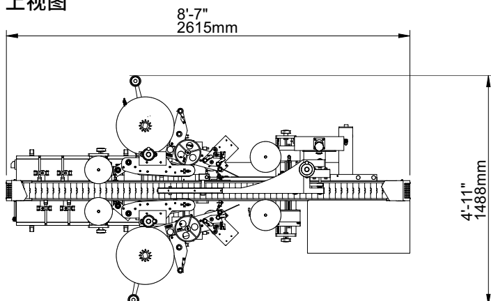
上视图
